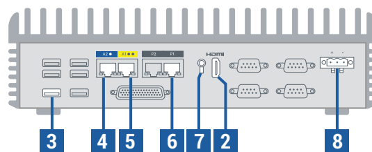
Família ztC Edge 100i (visão traseira)
