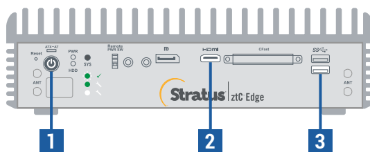
Família ztC Edge 100i (visão frontal)
