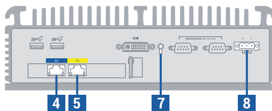
Família ztC Edge 110i (visão traseira)
