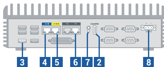
Família ztC Edge 100i (visão traseira)
