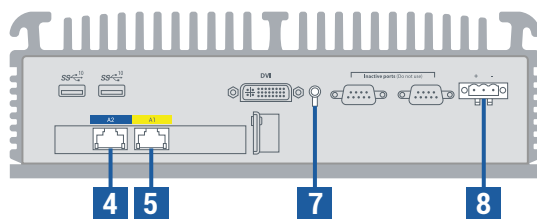
ztC Edge 110i 系列 (后视图)
