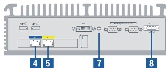
Sistemas ztC Edge 110i (visão traseira)
