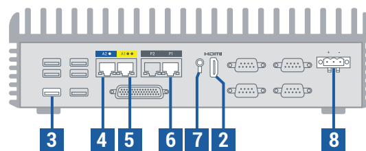
Sistemas ztC Edge 100i (visão traseira)
